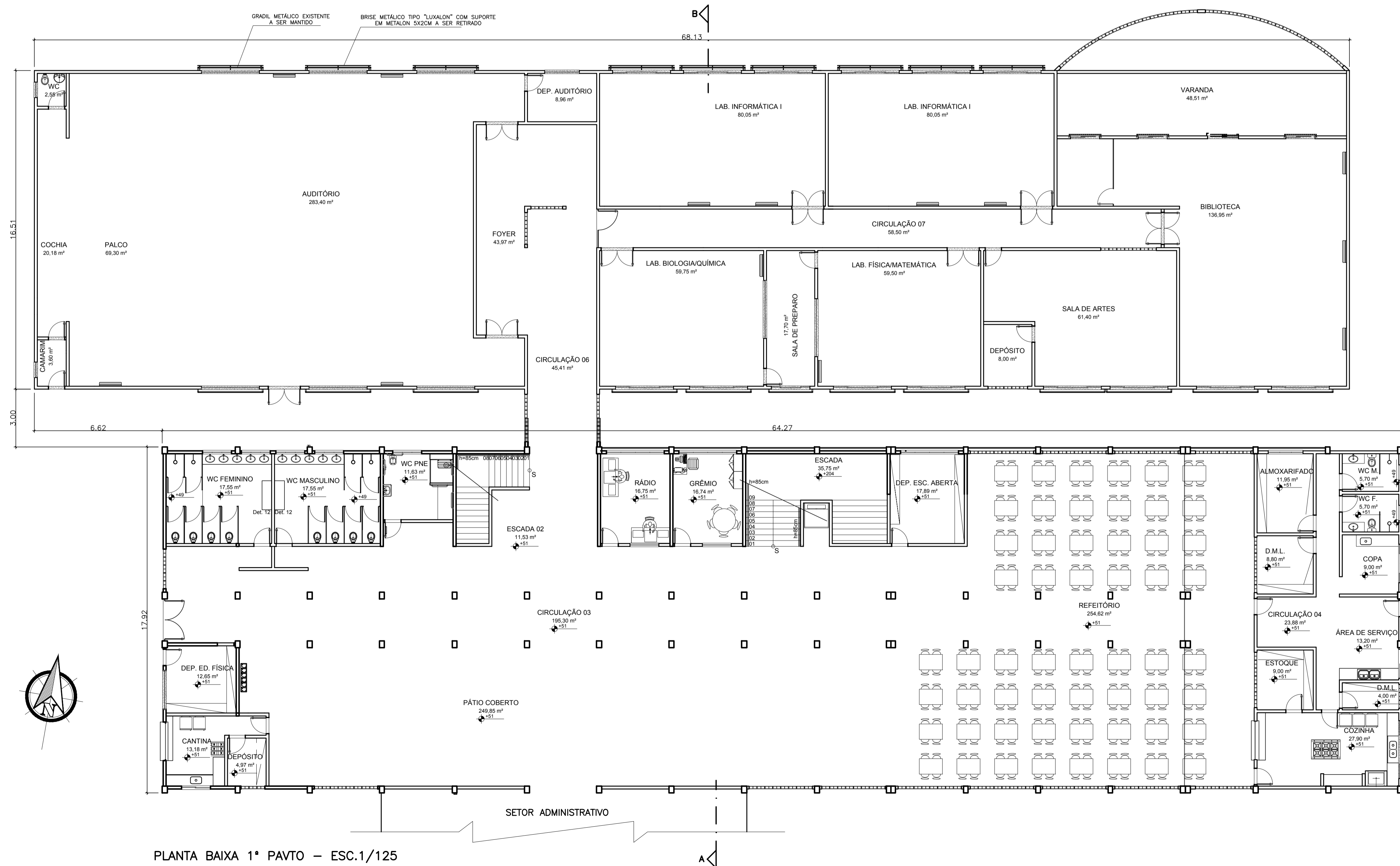
PLANTA BAIXA 2º PAVTO – ESC.1/125
